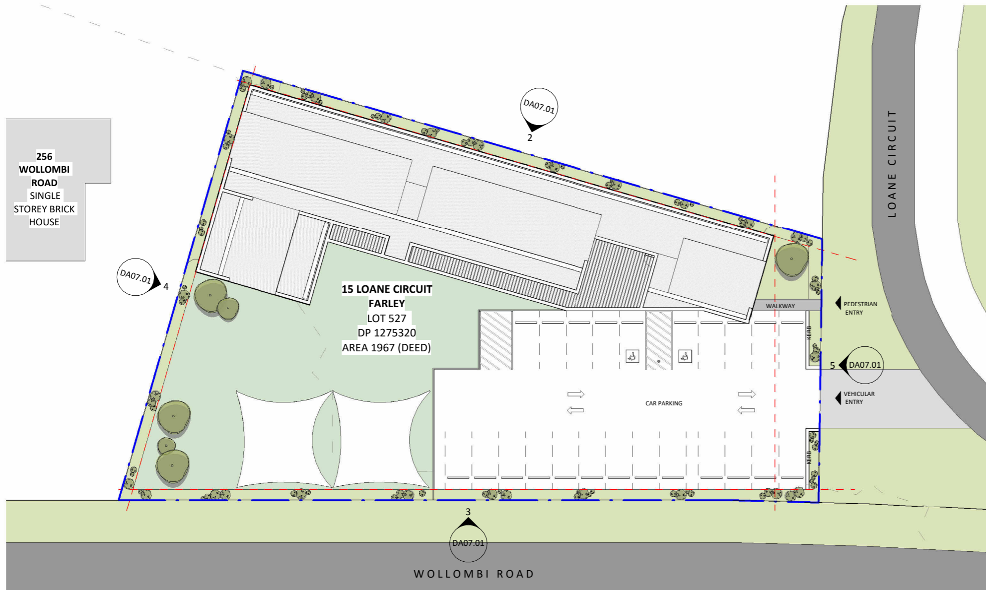
1 SITE PLAN 1:350
